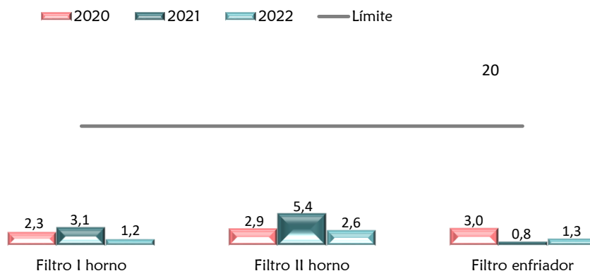
EMISIONES CONFINADAS DE PARTÍCULAS DE LOS PRINCIPALES FOCOS DE EMISIÓN DE LA PLANTA ( \text{mg}/\text{Nm}^3 )
